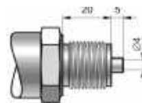
Тип М Штуцер M20x1,5 отверстие Ø4
