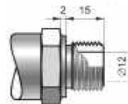
Тип Р Штуцер M20x1,5 отверстие Ø12
