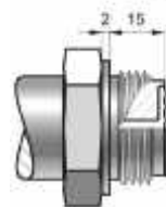
Тип SM30x2 10 кПа ≤ p < 7 МПа Штуцер M30x2 с лицевой мембраной Тип SM20x1,5 Штуцер M20x1,5 с лицевой мембраной; p ≥ 1 МПа
