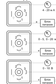
Рисунок 2 - Схема электрическая подключений преобразователей
