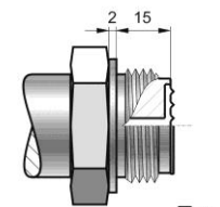
Тип CM30x2 10 кПа \leq p < 7 МПа Штуцер М30х2 с лицевой мембраной Тип CM20x1,5 Штуцер М20х1,5 с лицевой мембраной; p \geq 1 МПа
