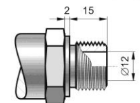
Тип Р Штуцер М20х1,5 отверстие \varnothing 12
