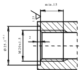
Рисунок Д.2б - Ответное гнездо для преобразователей с присоединением M20x1,5 типа Р с увеличенным отверстием
