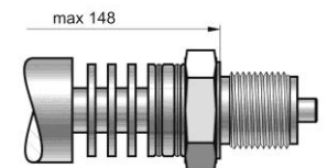
Тип RM 16 кПа \leq p < 4 МПа Радиатор с штуцером типа М Среда измерения с темп. до 150°С без импульсной трубки
