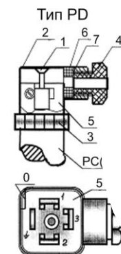
Рисунок 2 – Вид электрического присоединения
