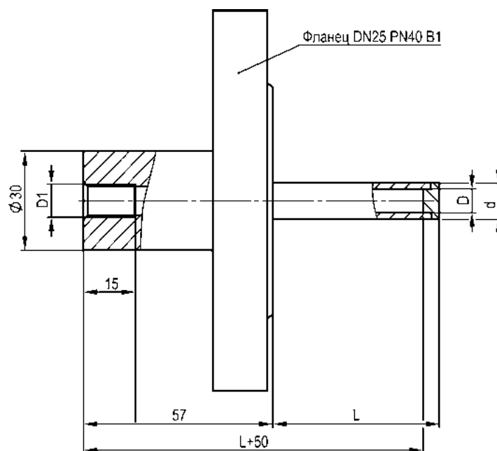
Рисунок 8 – Гильза цилиндрическая фланцевая ОТ1
