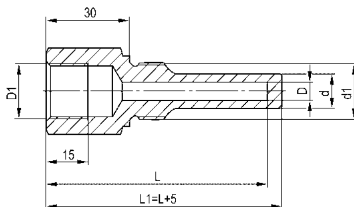
Рисунок 9 – Гильза цилиндрическая резьбовая цельноточеная OSWG1
