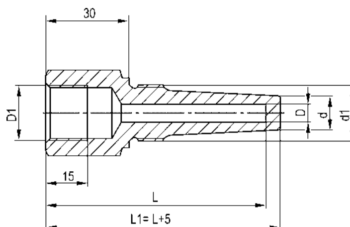
Рисунок 10 – Гильза коническая резьбовая цельноточеная OSWG2
