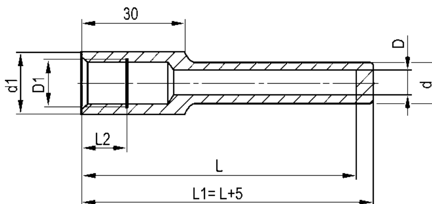
Рисунок 11 – Гильза цилиндрическая приварная цельноточеная OSW
