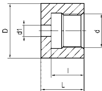
Рисунок 14 – Бобышка USM
