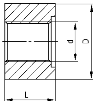
Рисунок 15 – Бобышка USP
