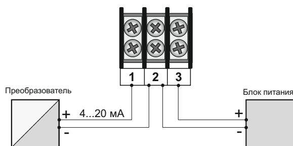
Схема электрических присоединений
