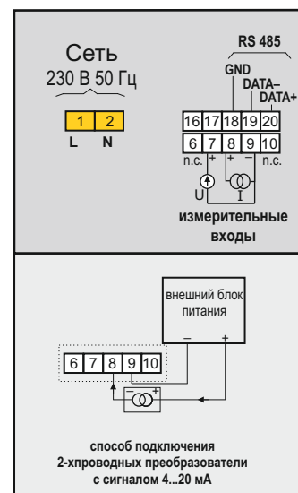
Схема электрических выводов
