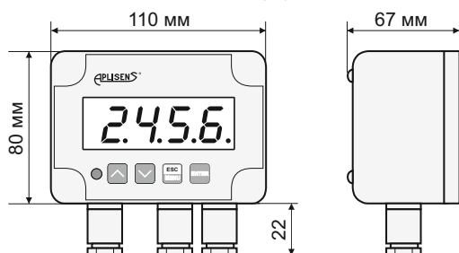
Степень защиты корпуса IP65
