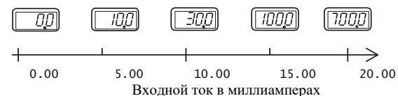
Рисунок 3 - Пример тарировки показаний измерителя для реализации нелинейной характеристики преобразования
