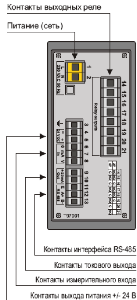
Рисунок Б.1 - Схема расположение контактов на задней панели измерителя-регулятора
